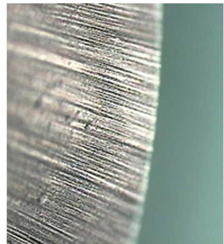
초경 스크라이버 휠 연삭 무늬
